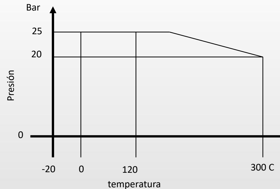
Grafica de presión vs temperatura
